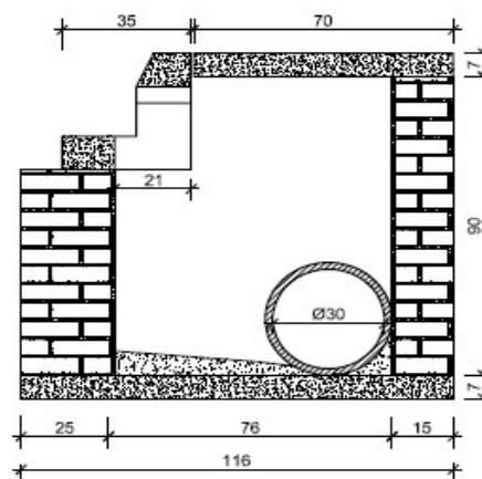
Boca de Lobo Padrão
