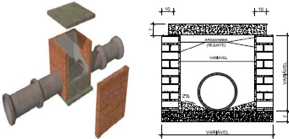
Poço de Visita Padrão no Passeio
