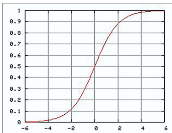
Figura 3.2: Curva Logística.
