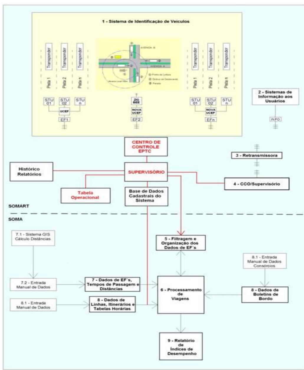
Figura 4 – Diagrama Funcional SOMA e SOMART
