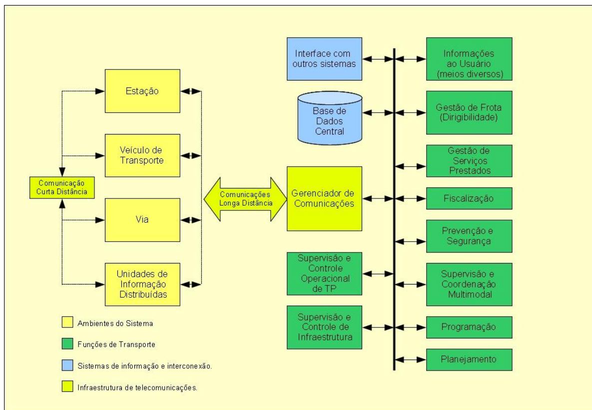
Figura 7 – Diagrama Funcional de ITS para Transportes
