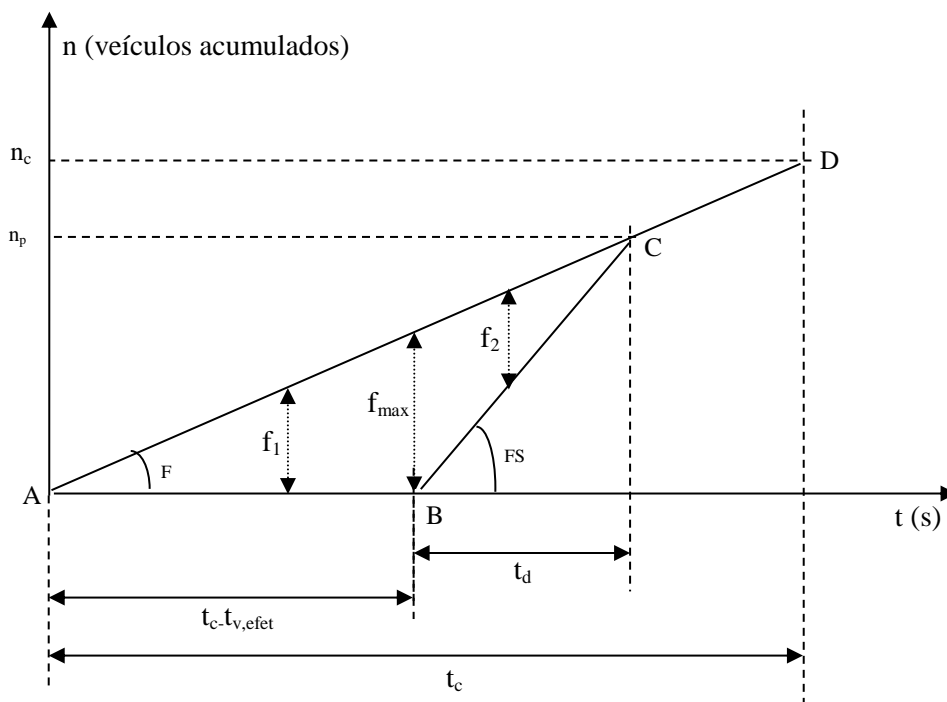
Figura 6.10: Processo de formação e dissipação de fila
