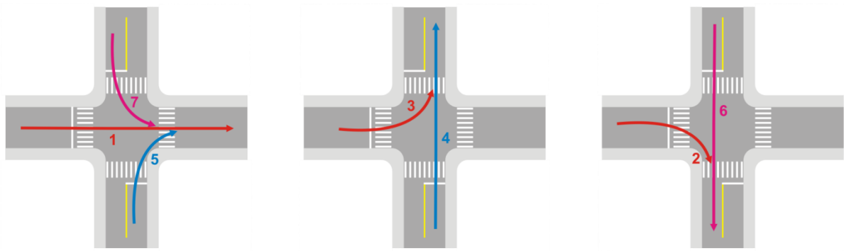
Figura 4.3: Movimentos convergentes
