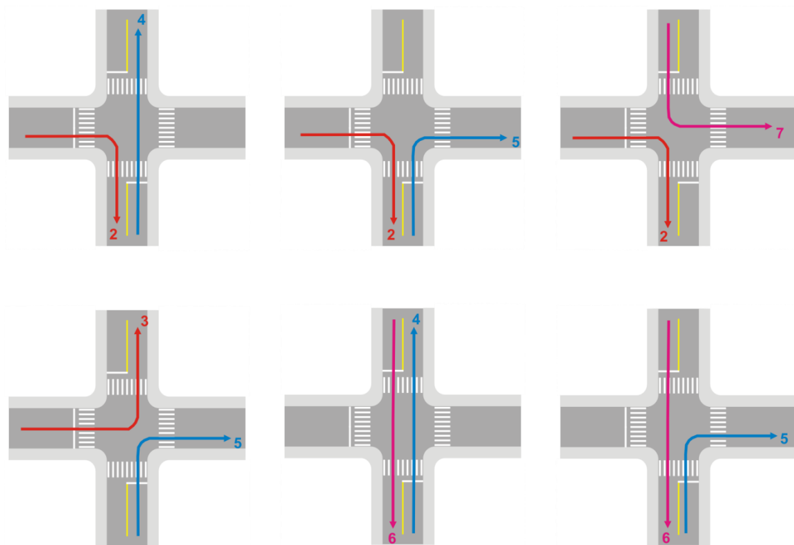
Figura 4.6: Movimentos não-interceptantes
