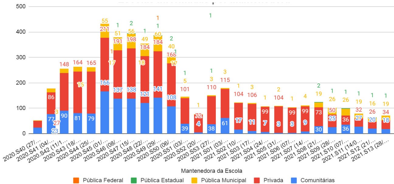
Gráfico 2 - Instituições de ensino por tipo de mantenedora
