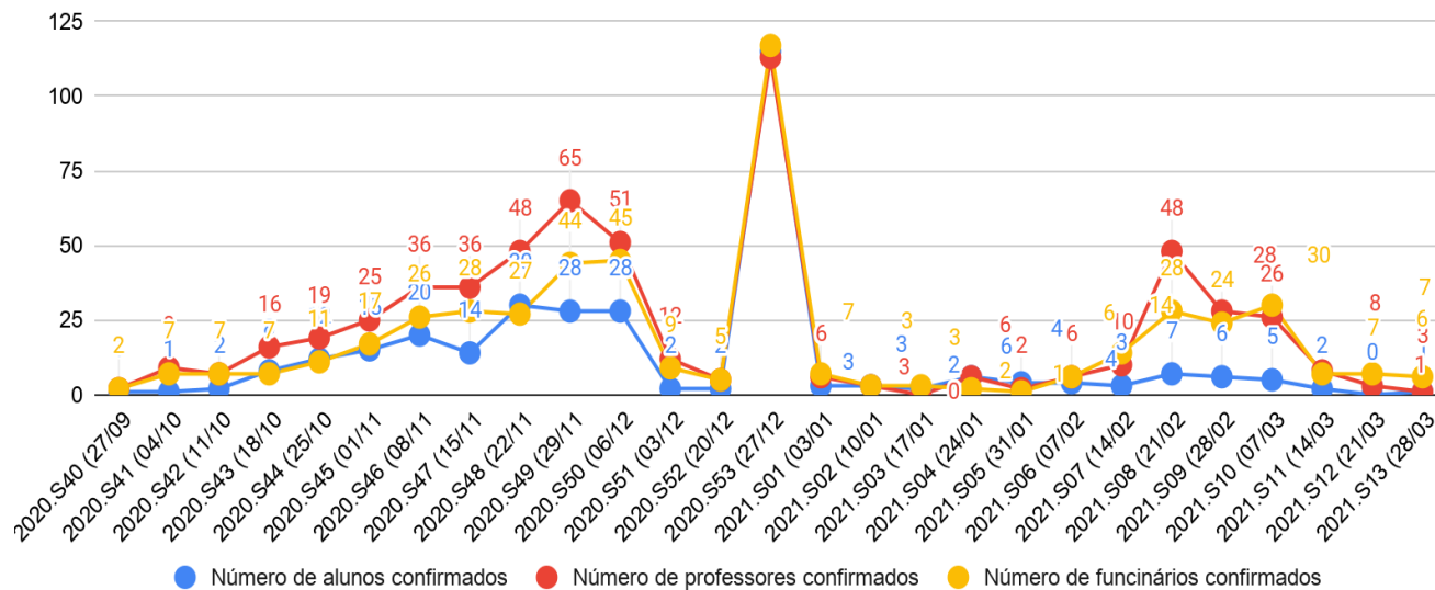
Gráfico 6 - Número de alunos, professores e funcionários com casos confirmados por semana epidemiológica
